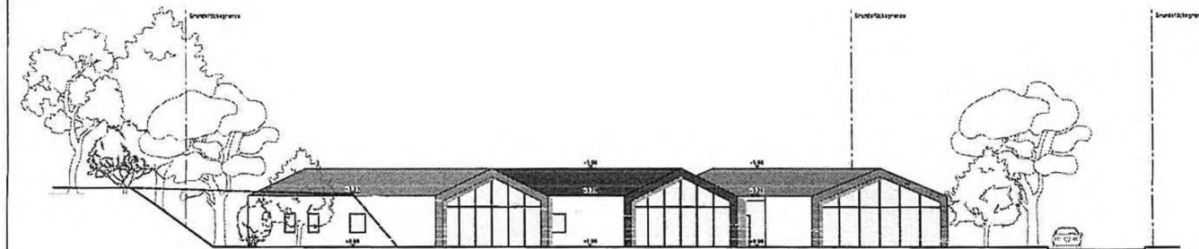
Ansicht Süd-West
